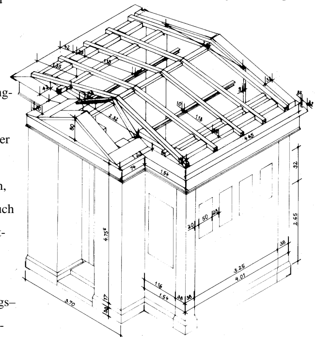
Friedhof II der Ev. Georgen-Parochialgemeinde Mausoleum Martiny, Konstruktionszeichnung
